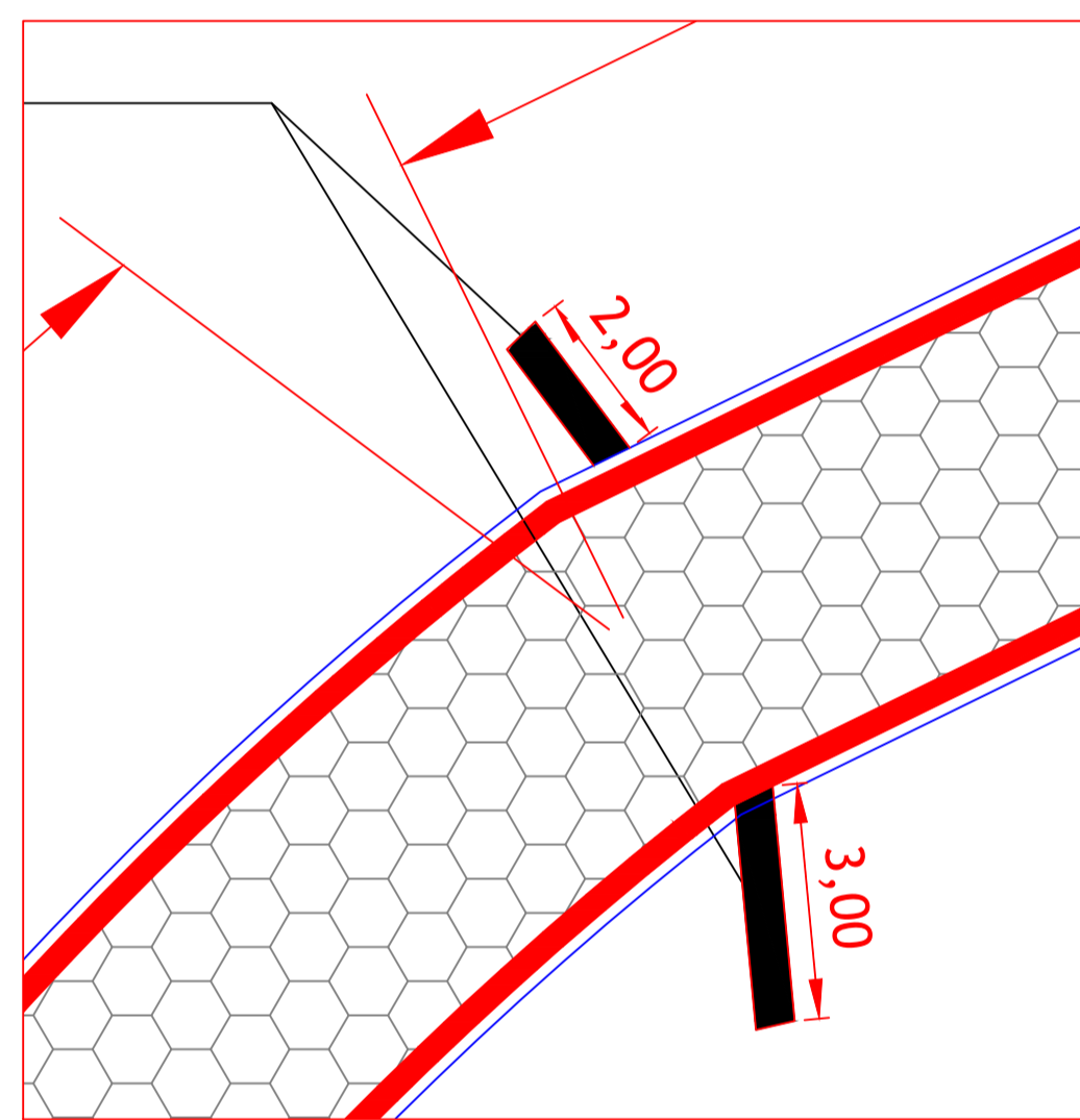
PLANTA EM CORTE DA RUA Sem escala
