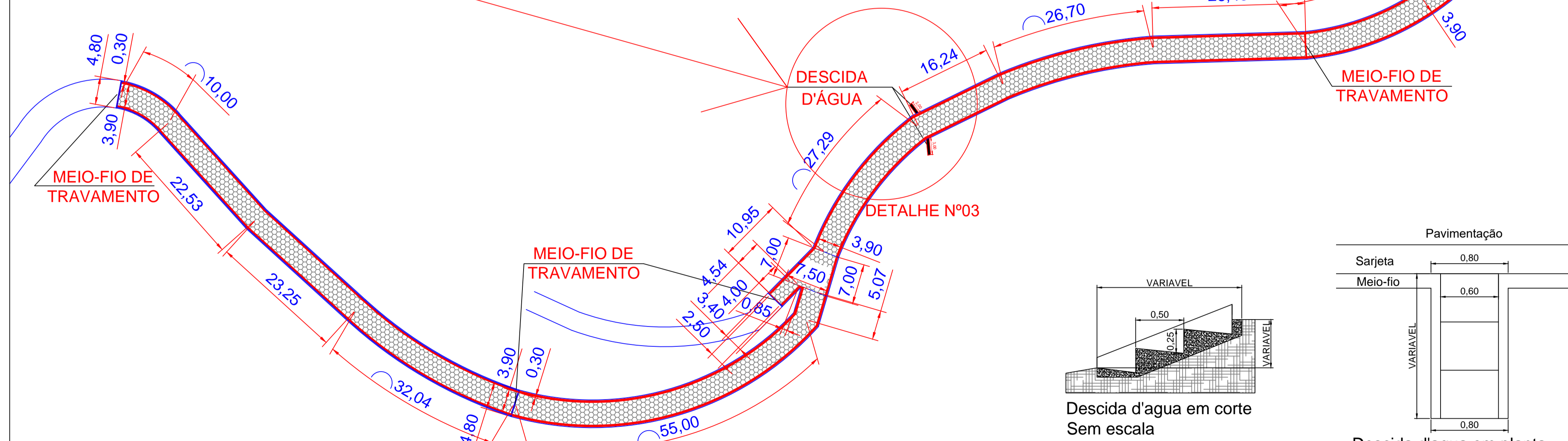
PLANTA TRECHO ESTRADA BAIRRO BREJINHO ESC: ..... 1:500
