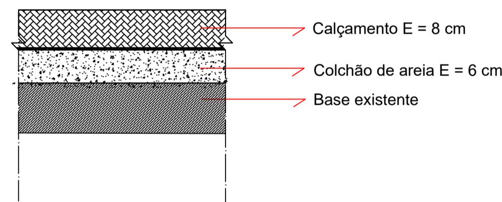
DETALHE Nº 1 Sem escala
